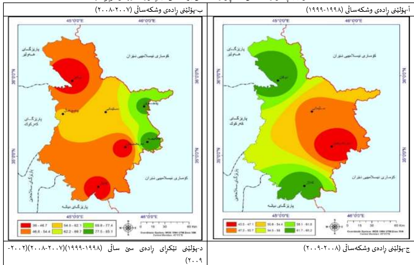
نه خشه ی (۲) رادهی و شکه سائی، تیکرای و شکه سائی بۆ سالیانی دیاریکراوی ناوچه ی توئینه وه
