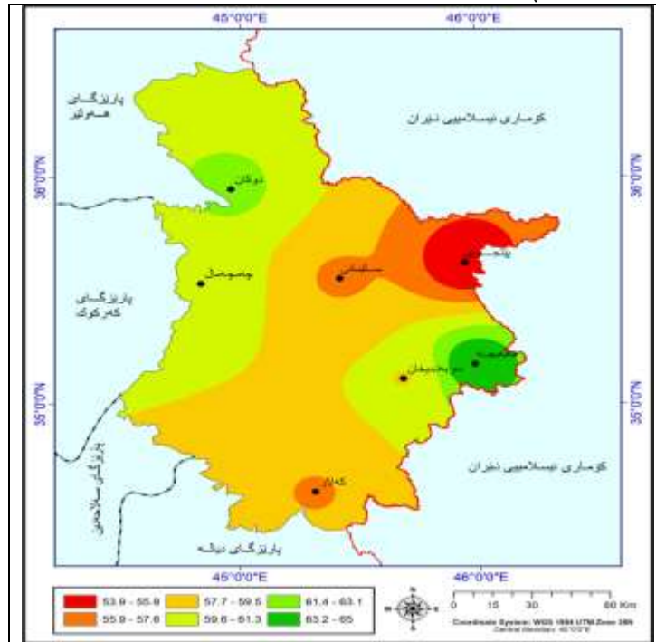
نەخشە (۳) تیکرای وشکەسائی لە پارێزگی سلیمانی و هەلەبجە لە ماوەی (۱۹۹۲-۲۰۱۸)
